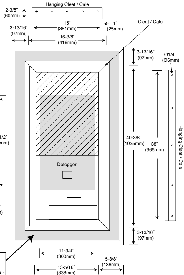
Back View / Vue arrière
