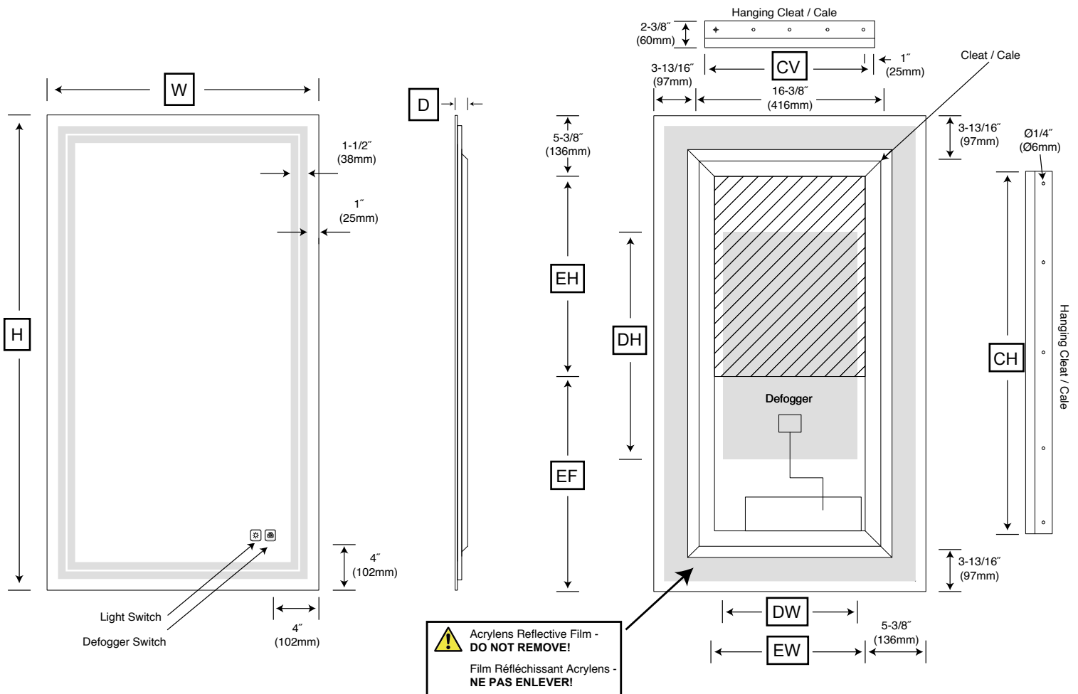
Front View / Vue de face
