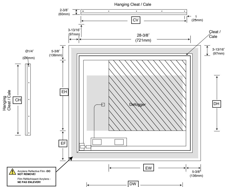
Back View / Vue arrière
