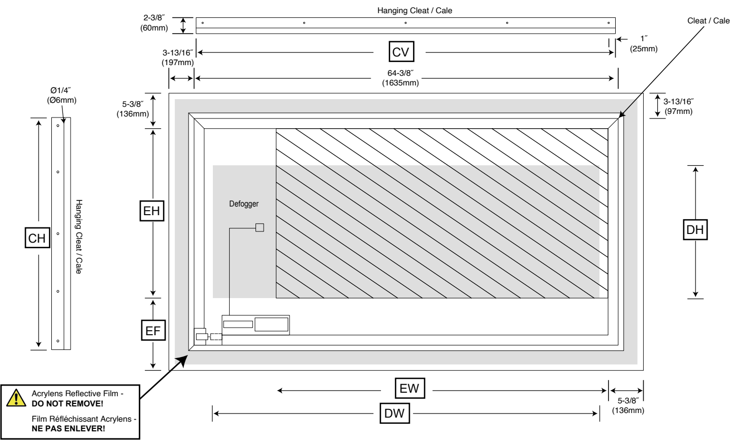
Back View / Vue arrière
